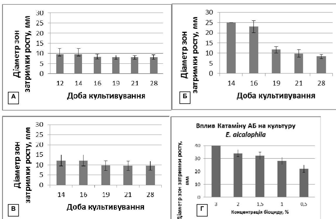
Рис. 1. Фунгістатичний вплив ефірних олій (А – Foeniculum vulgare , Б – Mentha piperita , В – Melaleuca alternifolia ) та біоцидний вплив бензалконію хлориду (Катаміну АБ) за різних концентрацій (Г) на E. alcalophila (20-а доба культивування)
